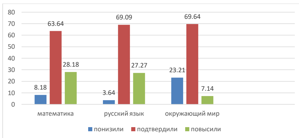
Сравнение отметок и результатов ВПР в 4 классах (в %)
